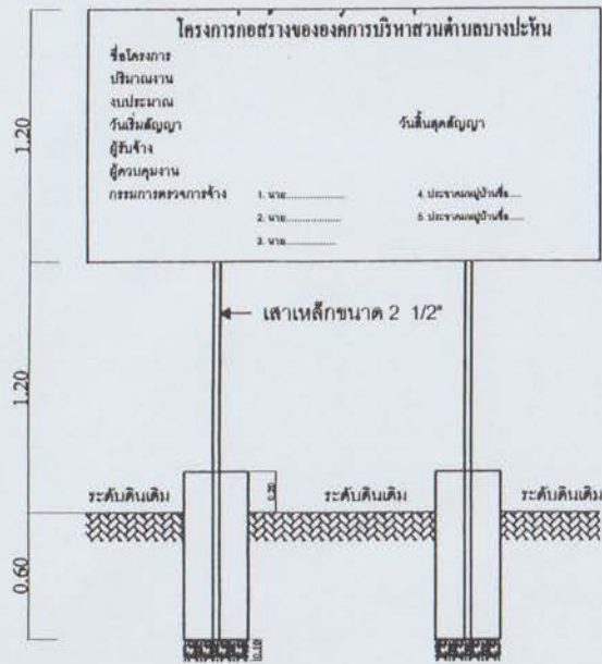
แบบป้ายโครงการ 1: 25
